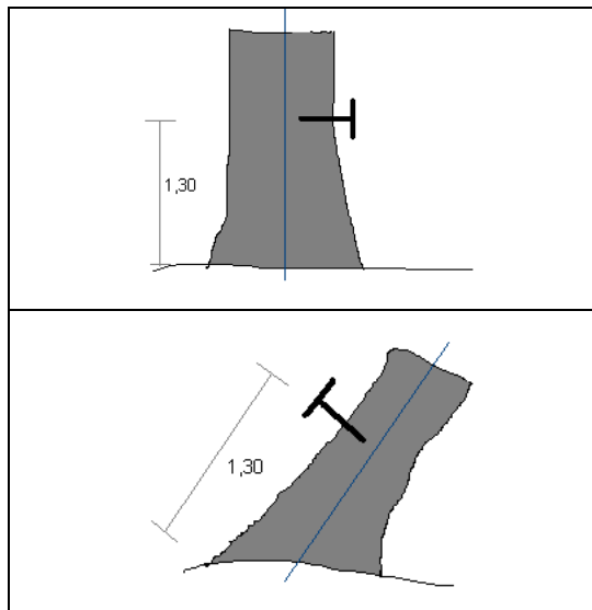
Figura 5.4.1 – Posizionamento e direzione della trivella per il prelievo della carota a 1.30 m.
