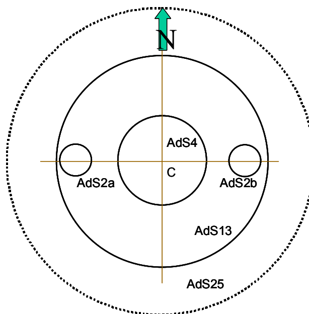
Figura 4.1 – Configurazione delle unità di campionamento di terza fase, con l'orientamento previsto nel caso di terreni pianeggianti.
