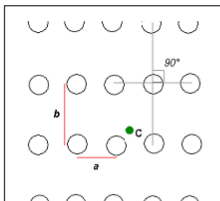
Figura 5.10.1b - Sesto rettangolare
