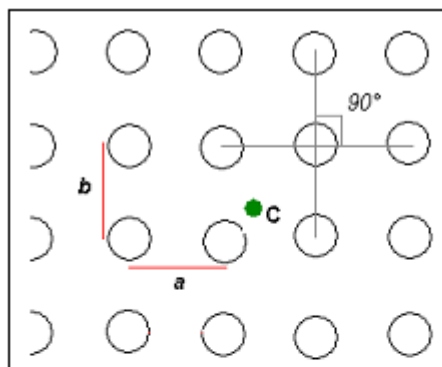
Figura 5.10.1a - Sesto quadrato
