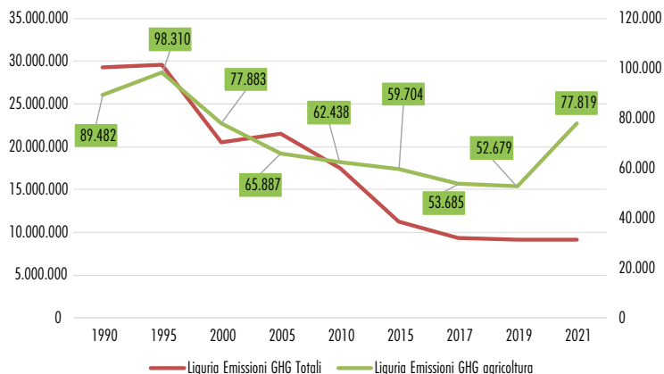
Andamento delle Emissioni di GAS Serra In Liguria 1990 - 2021 (t di CO 2 eq.)
